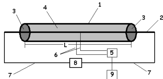
Figura 1. Esquema experimental, (1) tubo hueco (Incoloy 800), (2) varilla resistiva (NiCr 80-20), (3) tapones cerámicos, (4) muestra, (5) termómetro, (6) Termopares tipo K, (7) Conductor, (8) fuente variable ac (7V-300Amp.) y (9) computador PC.
