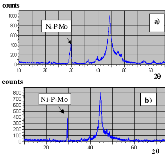
Figura 6. Espectro de difracción de rayos X del recubrimiento: a) a los 60 minutos, b) final al término de 180 minutos.
