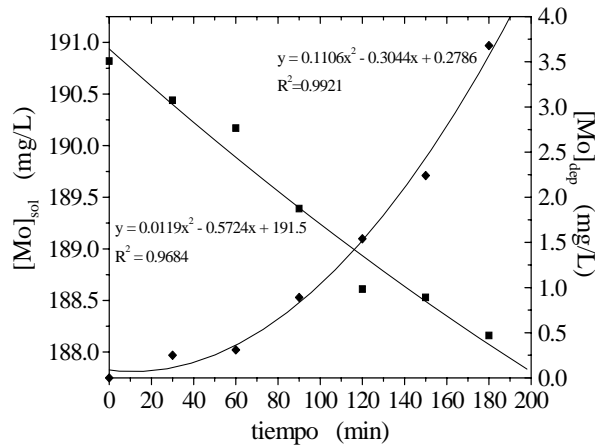
Figura 4 b). Comportamiento del Mo en disolución del baño de niquelado químico y en el depósito.
