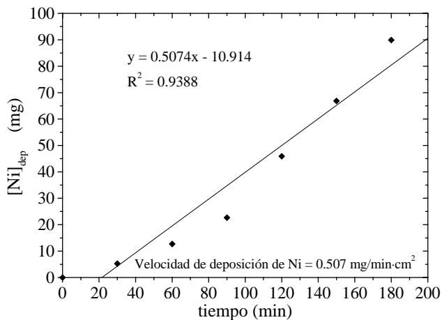
Figura 5 a). Velocidad de depósito del Ni.
