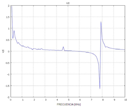
Figura 3. Impedancia de la cerámica piezoeléctrica al ser simulada.
