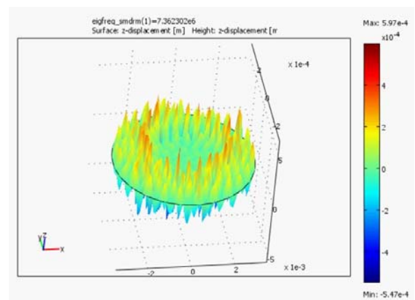
Figura 2. Simulación de la cerámica piezoeléctrica, mediante el método de los elementos finitos.
